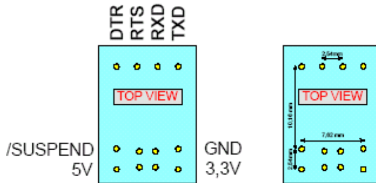
USB12 (Anschlußbelegung)
